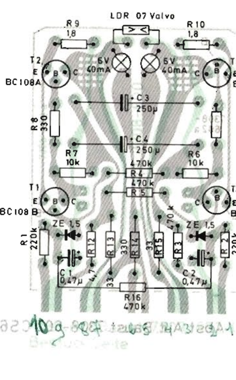
56 V-Platte, Lötseite 56 V PRINTED BOARD, SOLDER SIDE PLAQUETTE 56 V, VUE DU COTE DES SOUDURES PIASTRA 56 V, LATO SALDATURE
